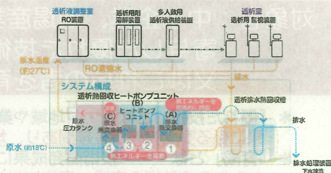
透析熱回収ヒートポンプシステム
