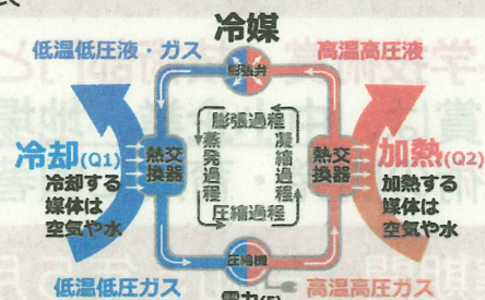
ヒートポンプの仕組み
